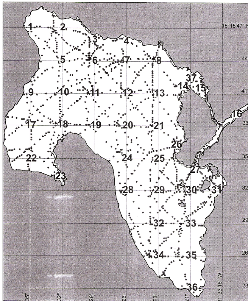
Fig. 3 – Répartition des 37 points remarquables et localisation des points bathymétriques mesurés dans la lagune de la Manche-à-Eau.
