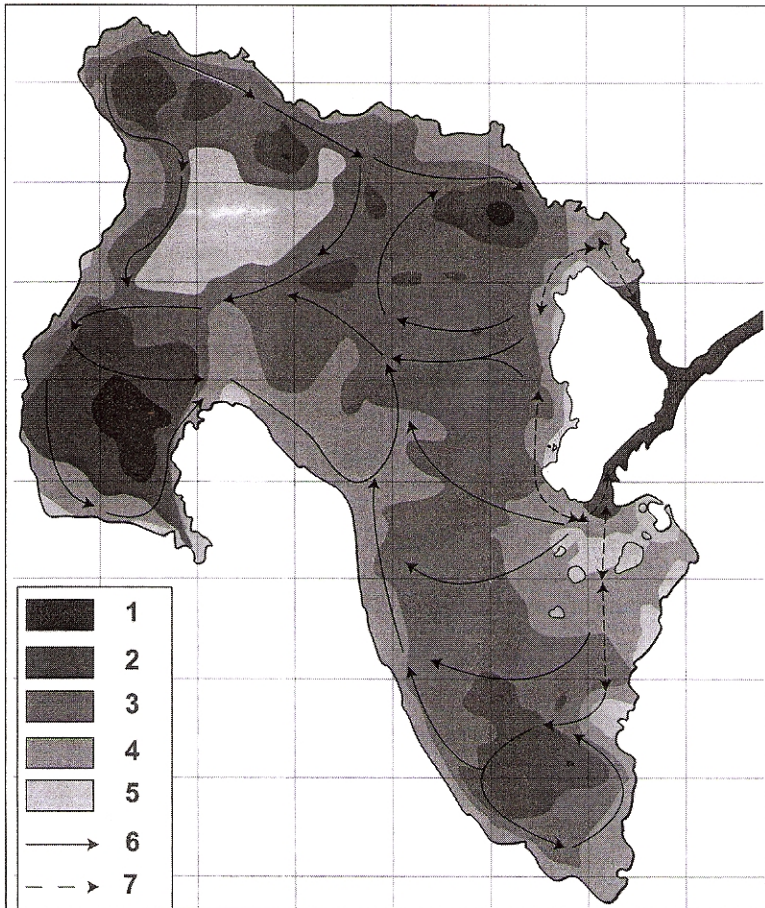
Fig. 5 – Courantologie et bathymétrie de la lagune de la Manche-à-Eau en 2007. 1 : [0 - 0,5[ m ; 2 : [0,6 - 1[ m ; 3 : [1,1 - 1,5[ m ; 4 : [1,6 - 2[ m ; 5 : [> 2] m ; 6 : circulation générale des courants ; 7 : courants de marée.
