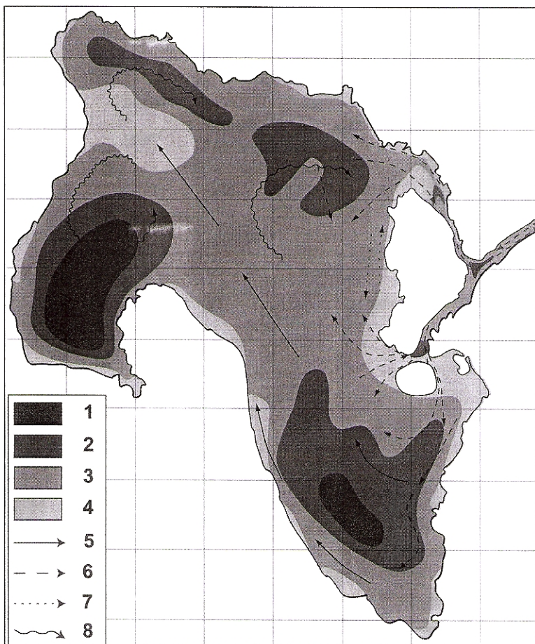
Fig. 6 – Courantologie et bathymétrie de la lagune de la Manche-à-Eau en 1987, d'après Assor. 1 : [0 - 1,5[ m ; 2 : [1,6 - 2[ m ; 3 : [2,1 - 2,5[ m ; 4 : [> 2,5] m ; 5 : circulation générale des courants en période de vent ; 6 : courants de marée ; 7 : courants alternatifs ; 8 : cellules tourbillonnaires.
